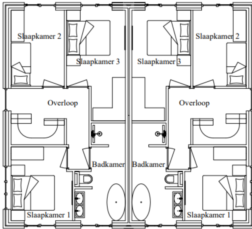
1e Verdieping
